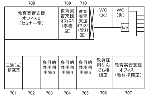
7 階 平 面 図
