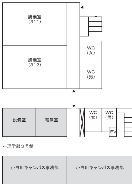
1 階 平 面 図
