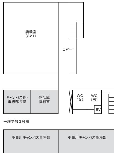
2 階 平 面 図
