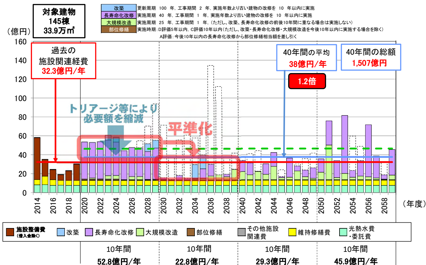
図 17 今後の維持・更新コスト (長寿命化型)
