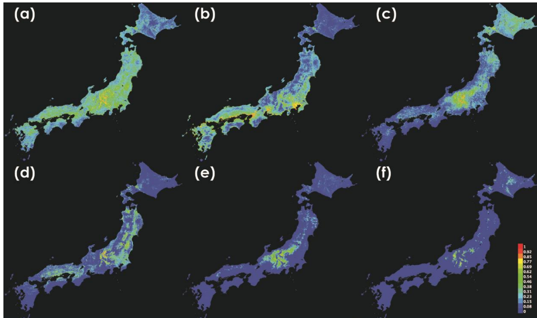
図 3： 6 種の生息地。赤いほど生息地である確率が高く、青いほど確率が低い。 (a) トラマルハナバチ、(b) コマルハナバチ、(c) オオマルハナバチ、 (d) クロマルハナバチ、(e) ミヤママルハナバチ、(f) ヒメマルハナバチ
