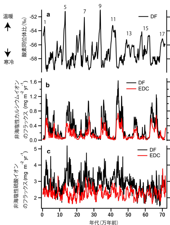
図3：過去72万年間を通じてのドームふじコアの酸素同位体比、および非海塩性カルシウムイオンと非海塩性硫酸イオンのフラックスの変動。ドームふじコア (DF) との比較のためにドームCコア (EDC) のデータも示す。酸素同位体比は気温変動の指標で、値が大きいほど温暖だったことを意味する。aに番号で示したのは、海底堆積物から決められた酸素同位体ステージであるが、ここでは間氷期のみ番号をつけた。非海塩性カルシウムイオンは、カルシウムイオンの総量から海塩起源のものを差し引いたもので、鉱物ダストの指標とされる。
