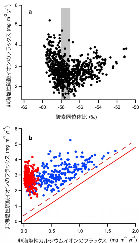
図4：ドームふじコアの非海塩性硫酸イオンのフラックスの変動。aは酸素同位体比との関係を、bは非海塩性カルシウムイオンのフラックスとの関係を示す。非海塩性硫酸イオンのフラックスはある酸素同位体比 (aのハッチをつけた部分)、つまりある気温を境に、それよりも温暖な時は気温の上昇とともに増加するが、それよりも寒冷な時は気温の低下とともに増加する。bの赤点は境目となる気温よりも温暖だったとき、青点は境目となる気温よりも寒冷だったときのデータ。寒冷だったときは、非海塩性硫酸イオンと非海塩性カルシウムイオンの相関が高い。
